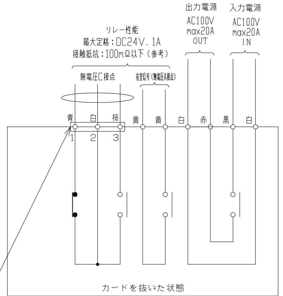
回路図
